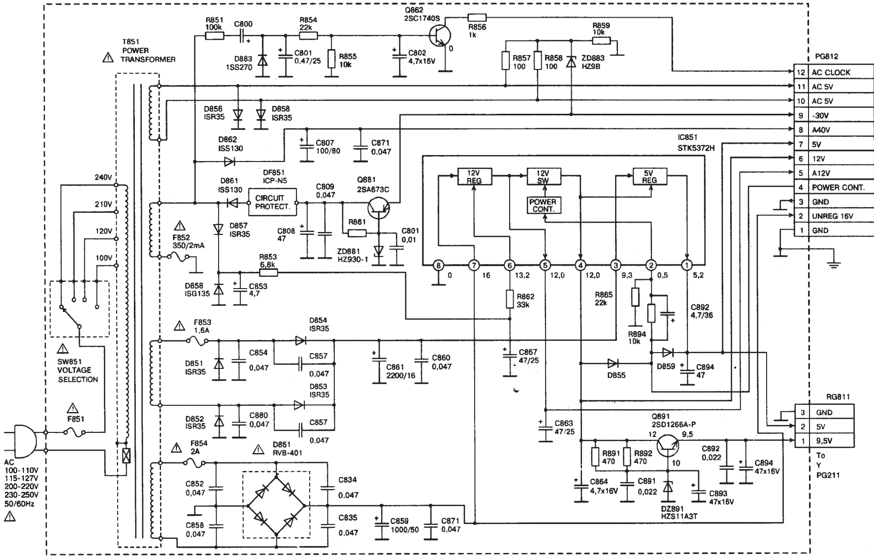
Принципиальная схема источника питания видеомэагнитофона VT-498EM
